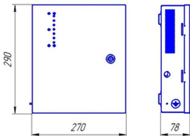
Рисунок 2 – Габаритные размеры трансляционного аудиоусилителя STS-301U
