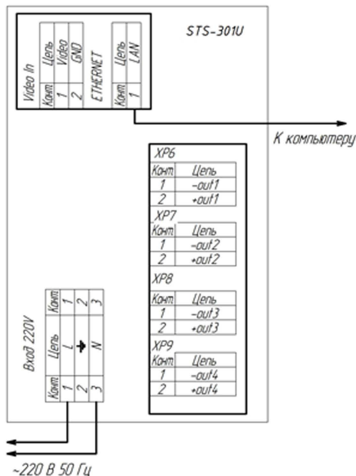
Рисунок 4 – Схема подключения блока к компьютеру
