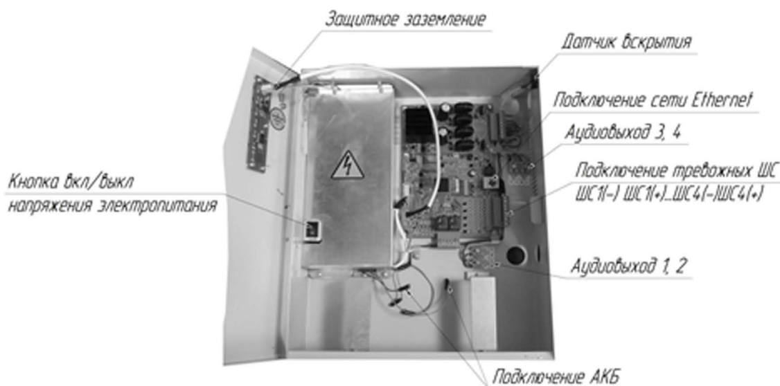
Рисунок 3 – Расположение составных частей и места подключений изделия
