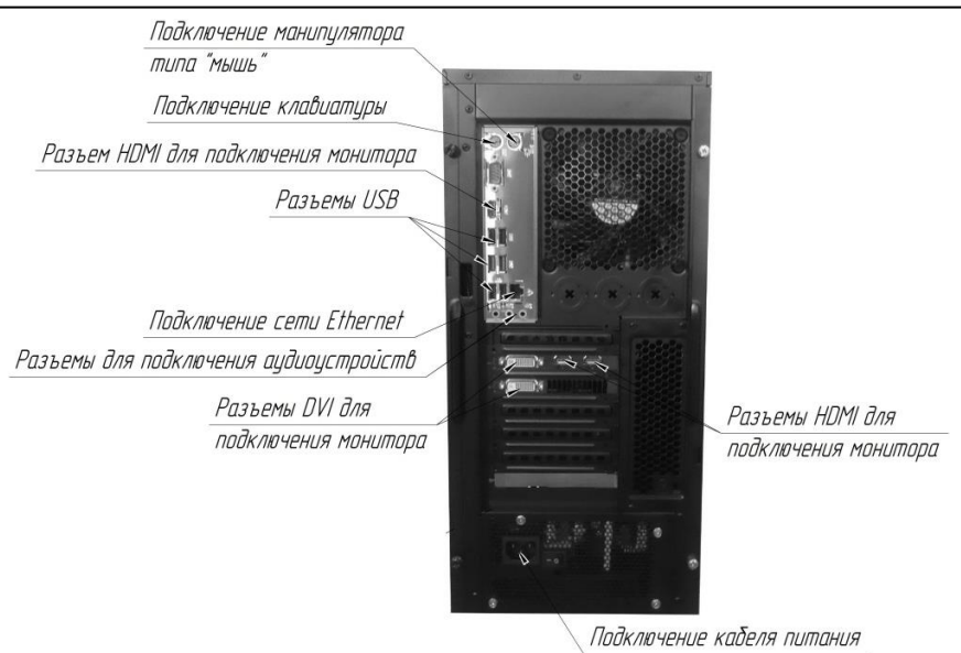
Рисунок 1 – Подключение системного блока (расположение и внешний вид разъемов может отличаться от приведенного)
