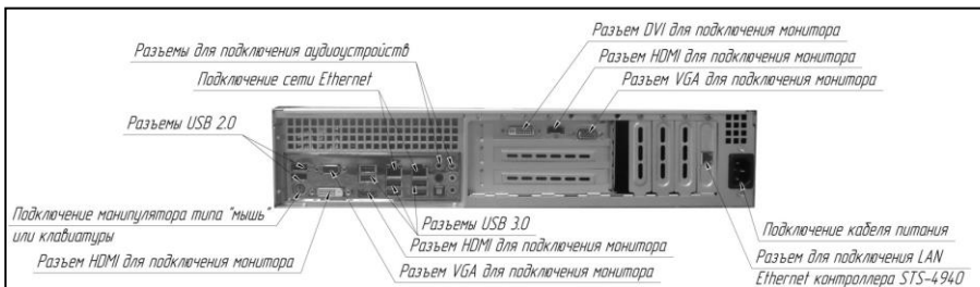
Рисунок 1 – Подключение сервера (внешний вид может отличаться от приведенного)
