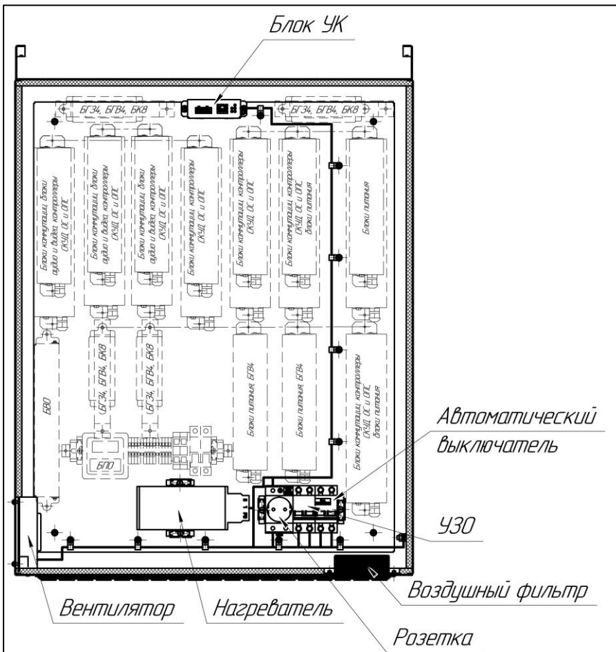
Рисунок 1 – Размещение блоков на монтажной панели
