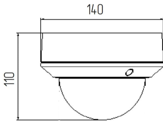
Рисунок 2 – Габаритные размеры изделия TBS-VS
