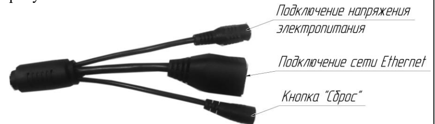
Рисунок 1 – Подключение IP-видеокамеры
