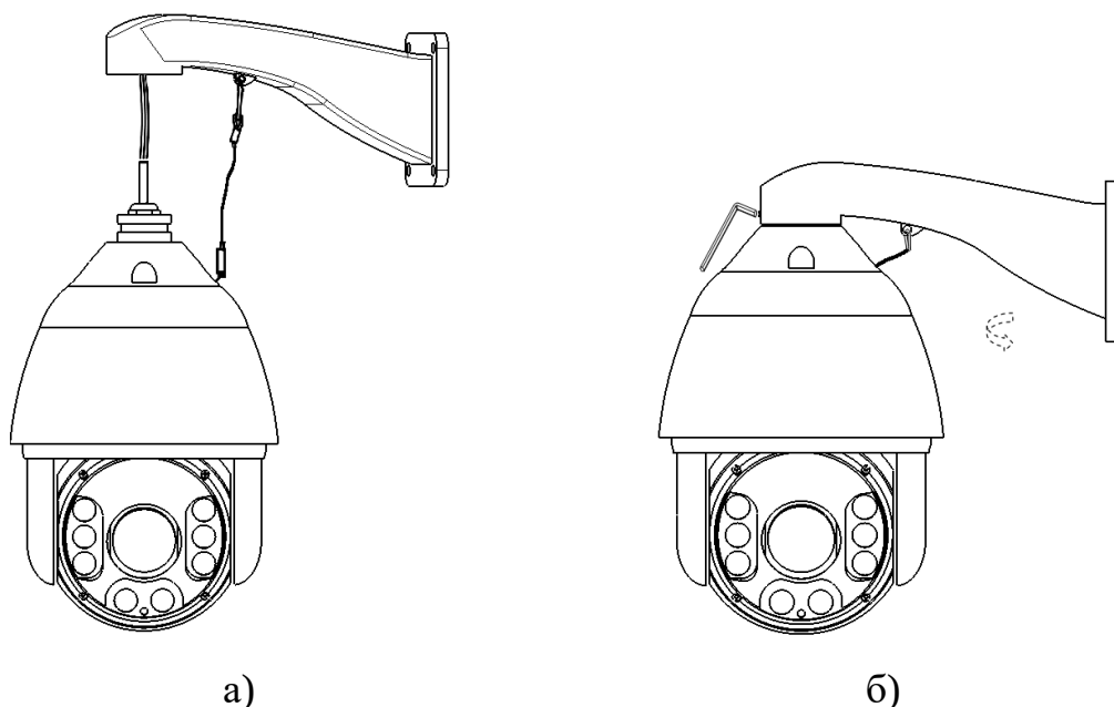
Рисунок 6 - Установка видеокамеры на кронштейне
