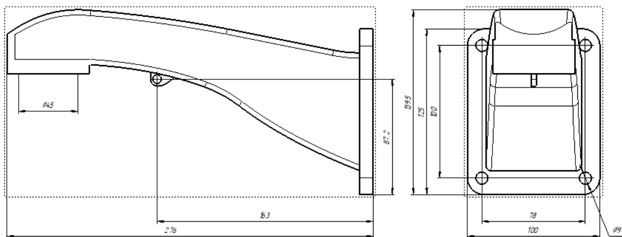
Рисунок 3 – Габаритные размеры кронштейна IP-видеокамеры SDP-850
