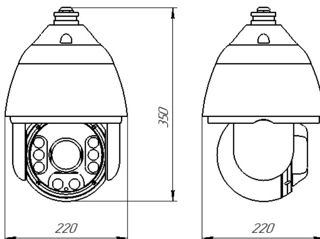
Рисунок 2 – Габаритные размеры изделия
