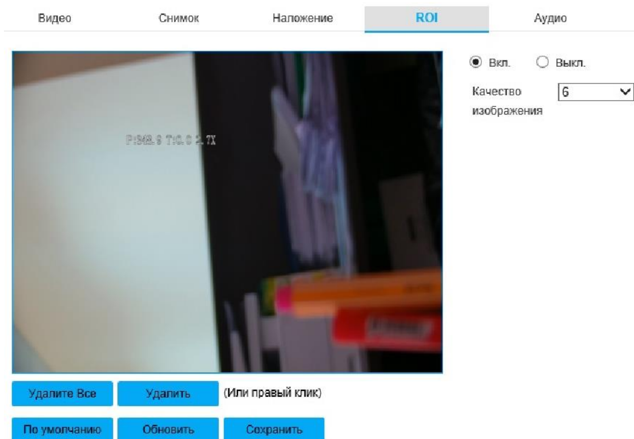
Рисунок 29 - Вкладка «ROI»
