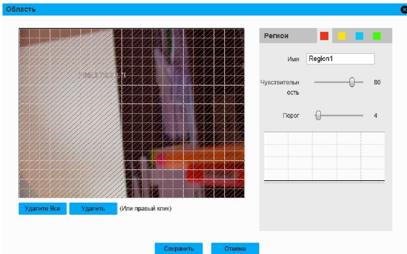
Рисунок 62-Вкладка «Область»
