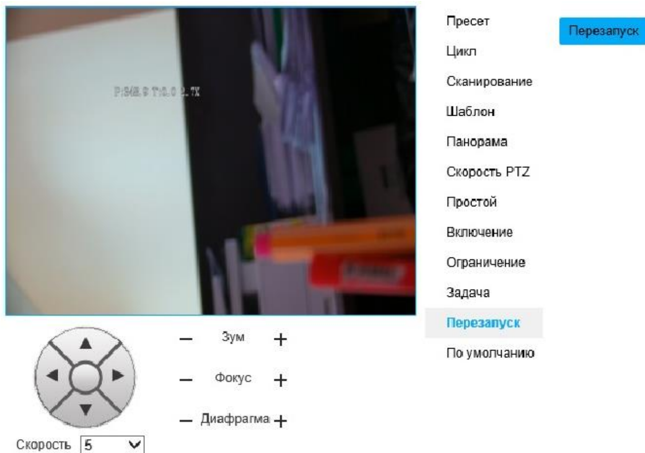
Рисунок 58 - Вкладка «Перезапуск»
