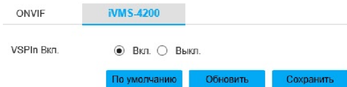
Рисунок 46 - Вкладка «iVMS-4200»
