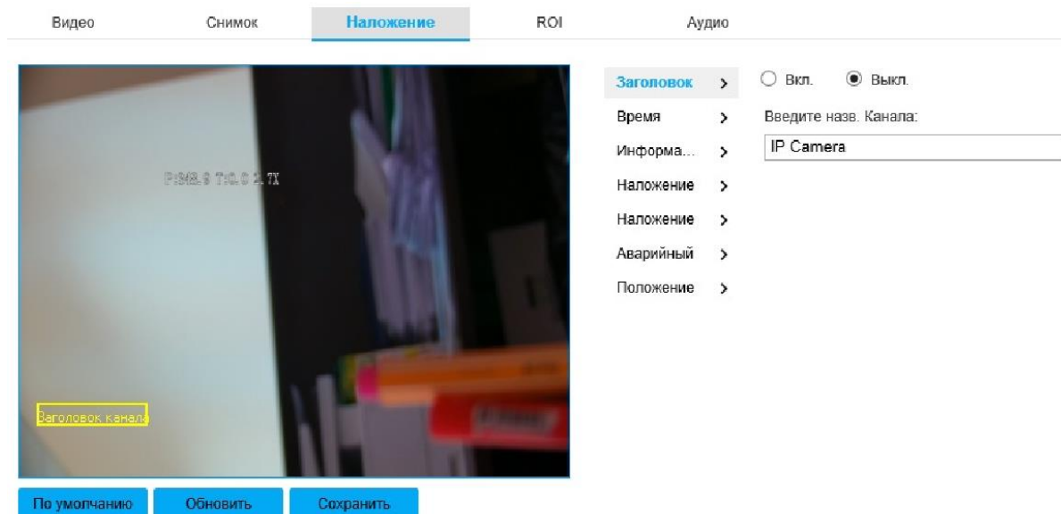
Рисунок 22 - Вкладка «Наложение»
