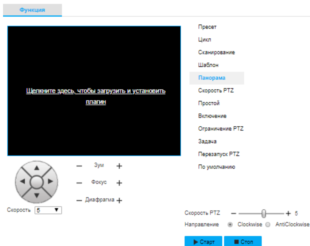
Рисунок 52 - Вкладка «Панорама»
