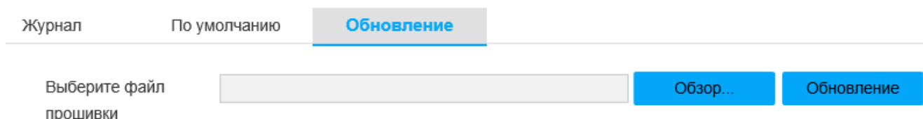
Рисунок 105 - Вкладка «Обновление»
