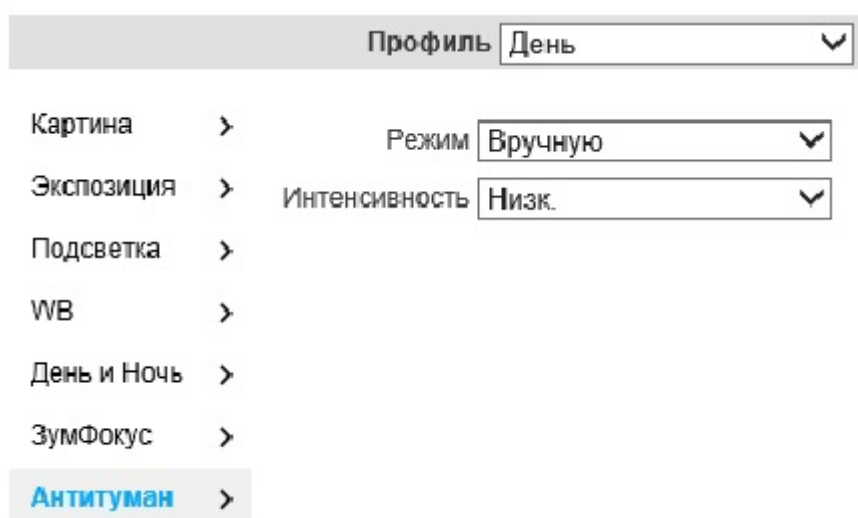
Рисунок 18 - Вкладка «Антитуман»
