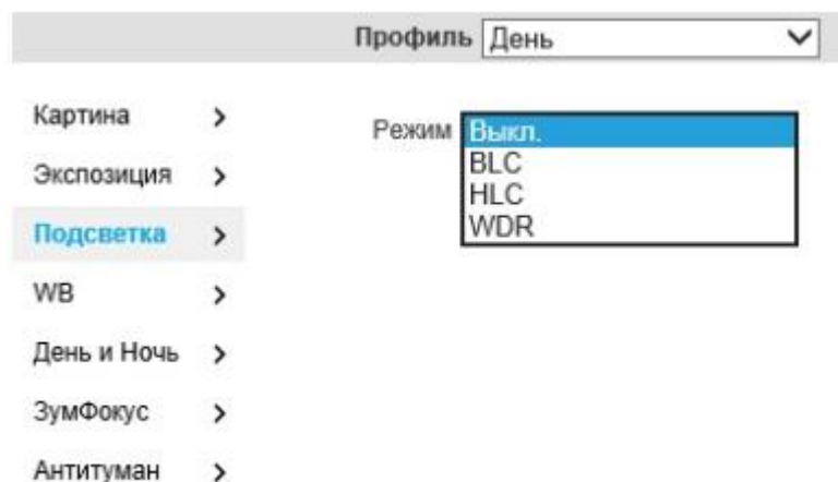
Рисунок 14 - Вкладка «Подсветка»
