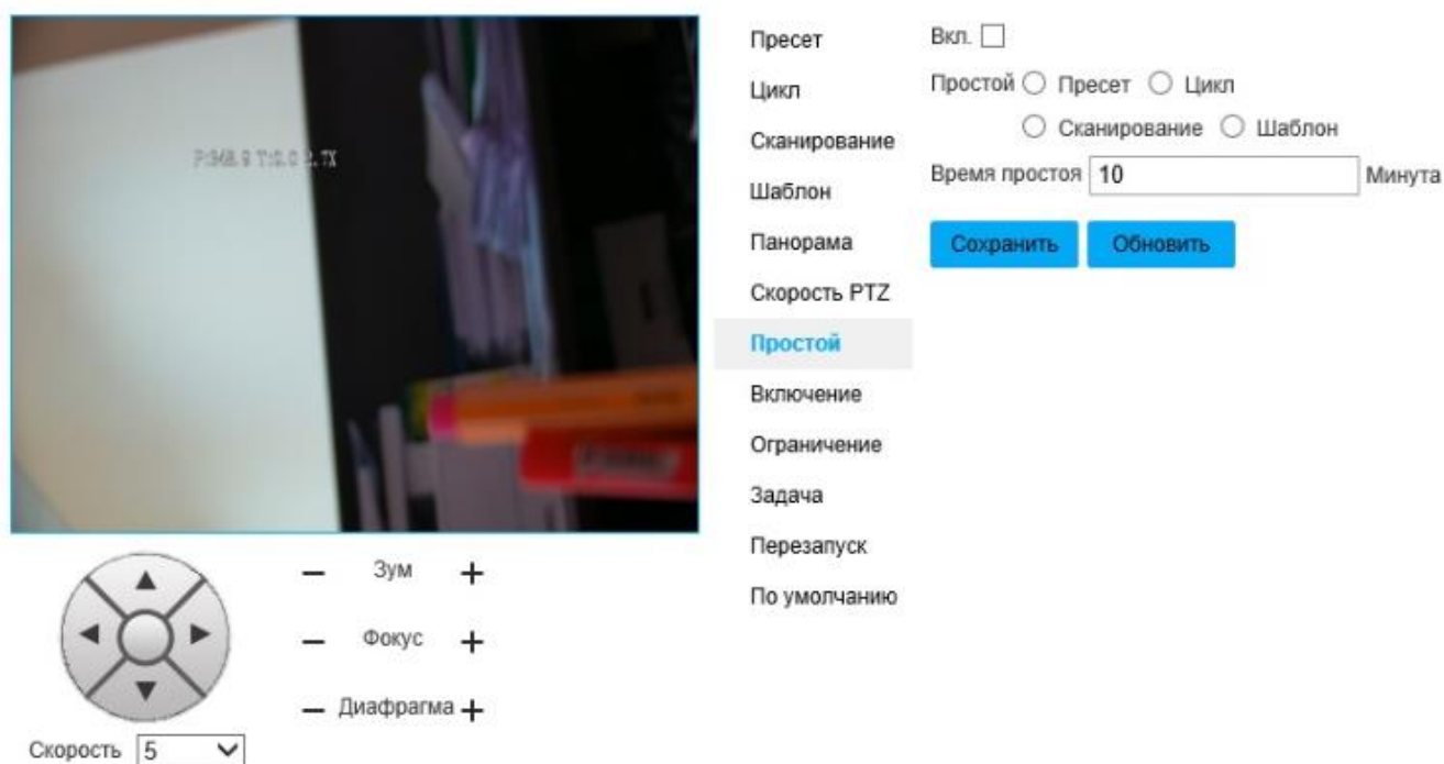
Рисунок 54 - Вкладка «Простой»
