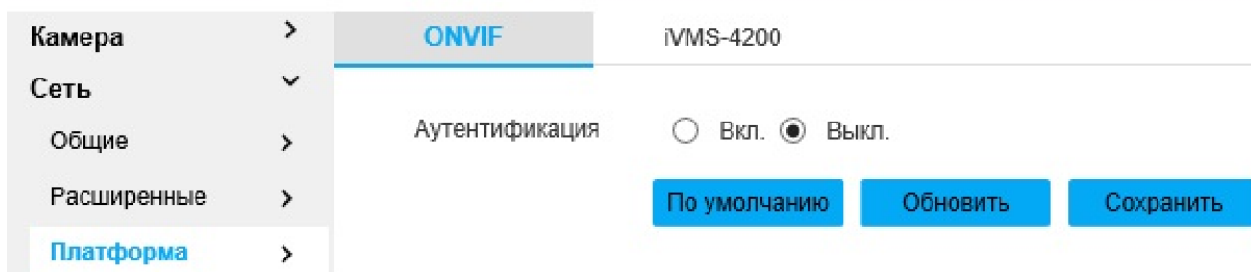
Рисунок 45 - Вкладка «Платформа»
