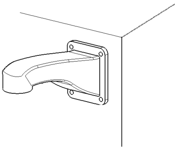
Рисунок 5 - Подготовка и установка кронштейна на стену
