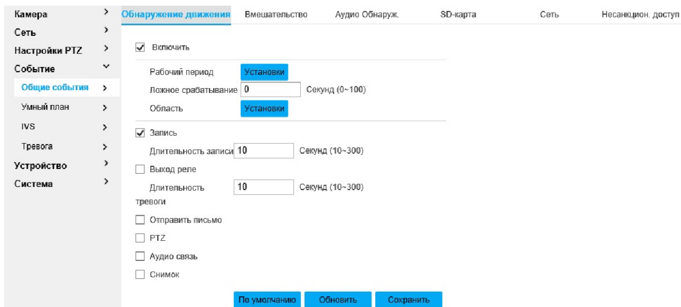
Рисунок 63- Вкладка «Вмешательство»
