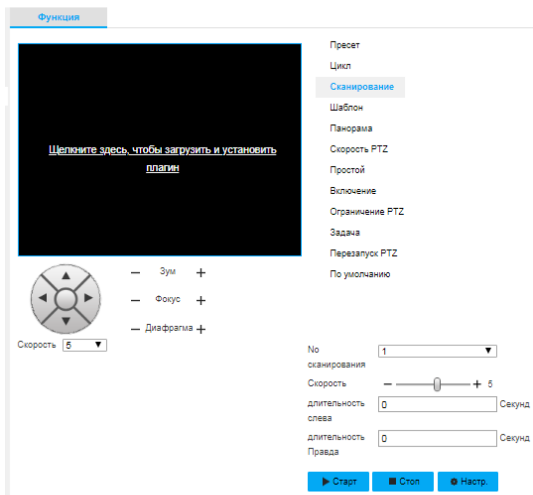
Рисунок 50 - Вкладка «Сканирование»
