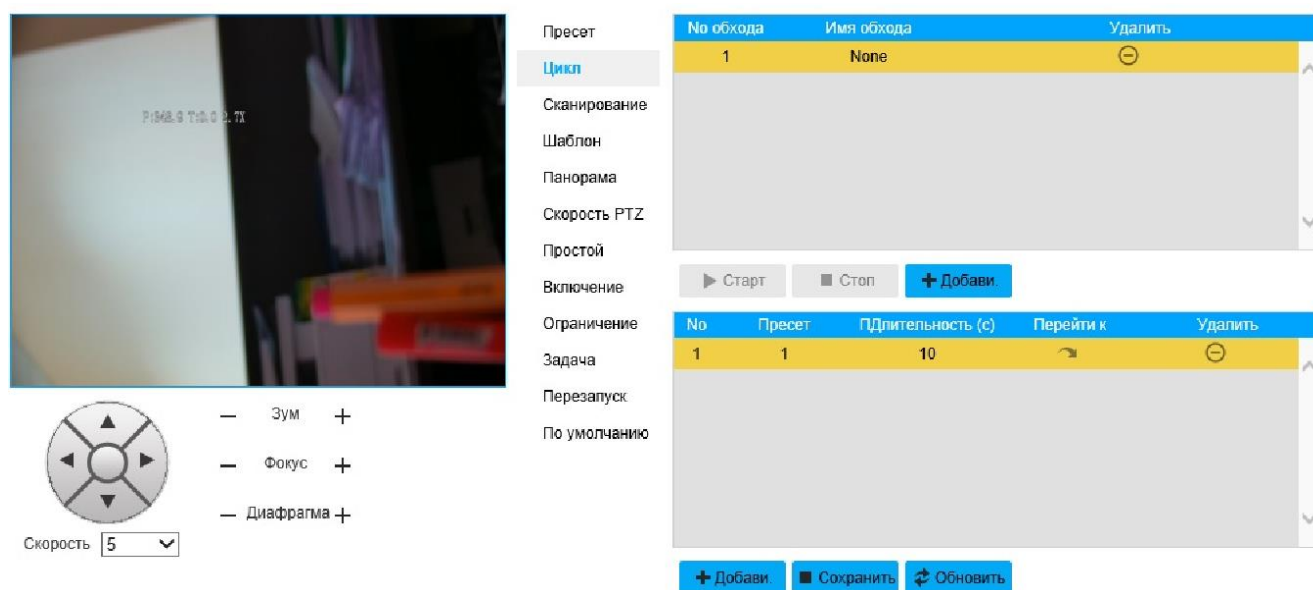
Рисунок 49 - Вкладка «Цикл»
