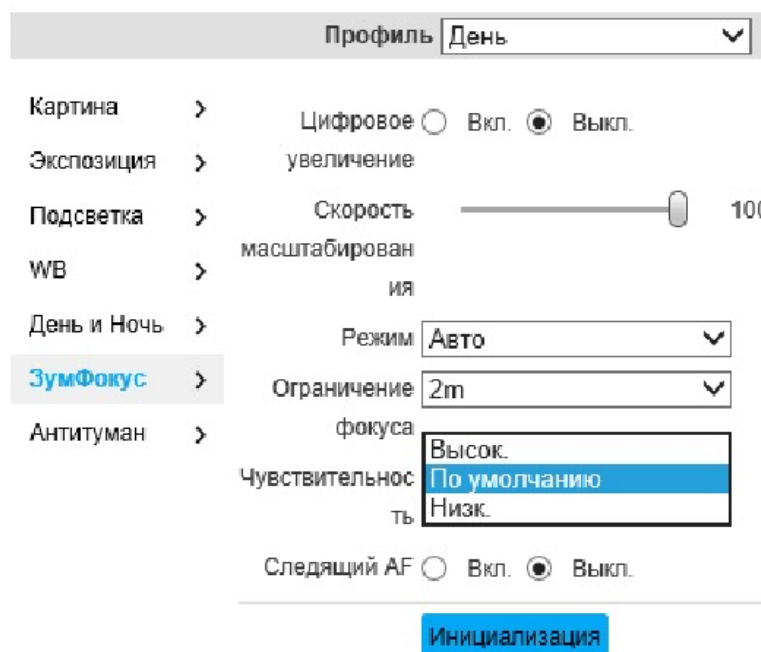
Рисунок 17 - Вкладка «ЗумФокус»
