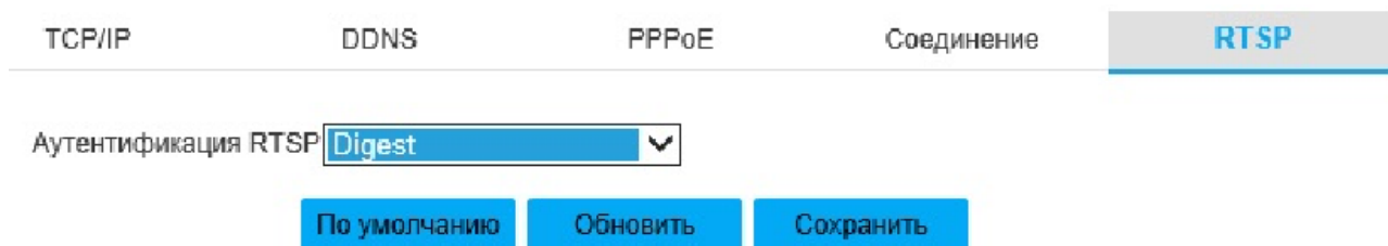
Рисунок 35- Вкладка «RTSP»
