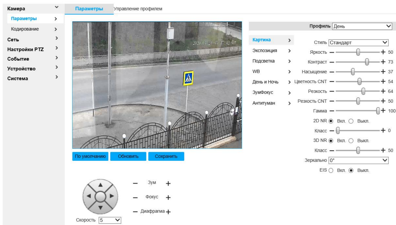
Рисунок 12 - Вкладка «Параметры»
