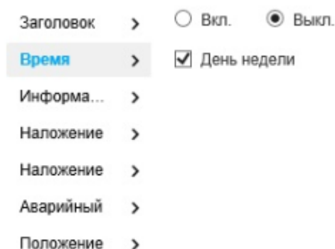
Рисунок 23 - Подкладка «Время»
