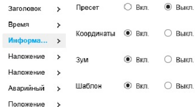
Рисунок 24 - Подкладка «Информация»
