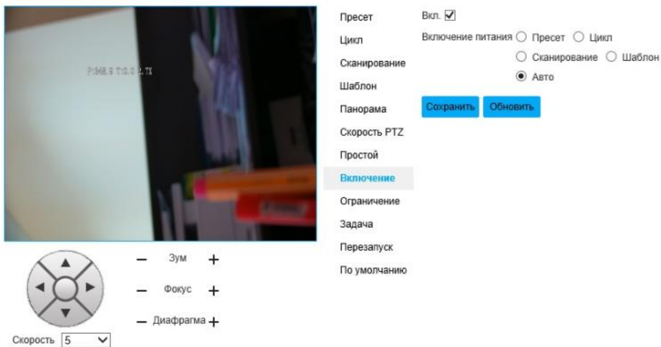
Рисунок 55 - Вкладка «Включение»
