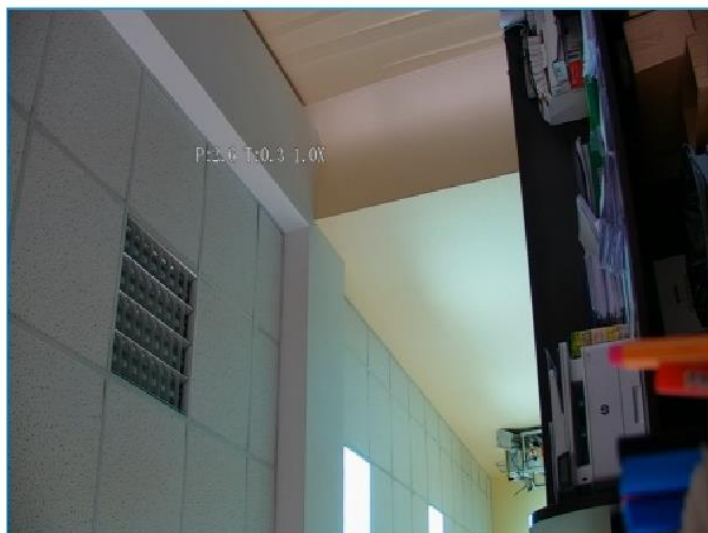
Рисунок 69 - Вкладка «IVS»
