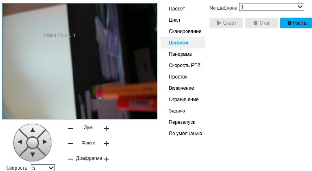
Рисунок 51 - Вкладка «Шаблон»
