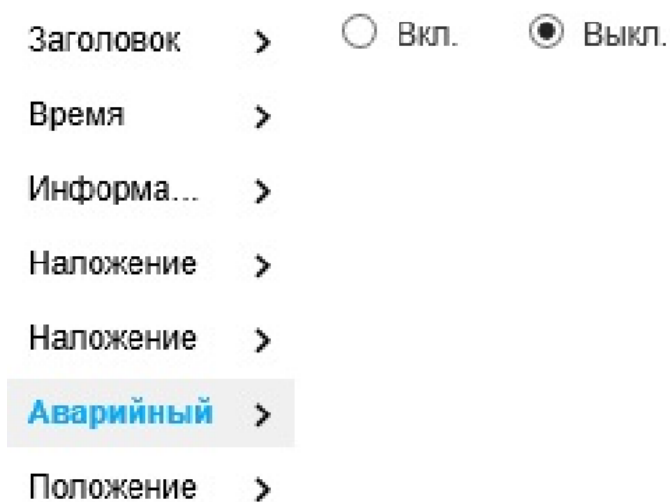
Рисунок 27 - Подвкладка «Аварийный»
