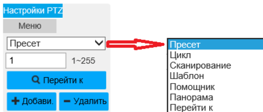
Рисунок 10 - Настройки PTZ
