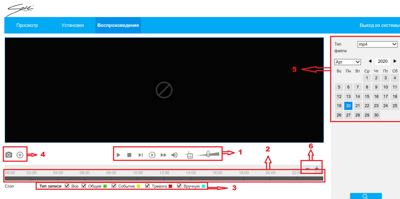
Рисунок 106 - Вкладка «Воспроизведение»
