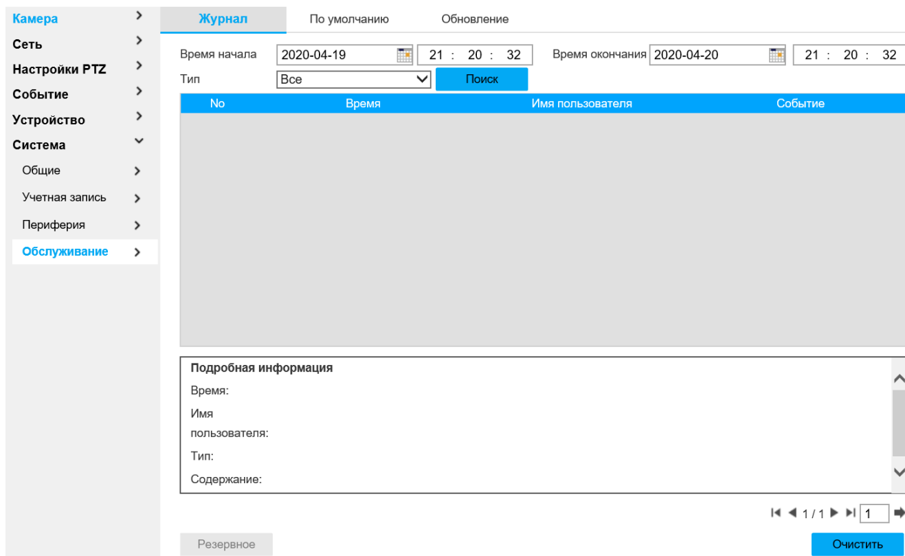
Рисунок 103-Вкладка «Обслуживание»
