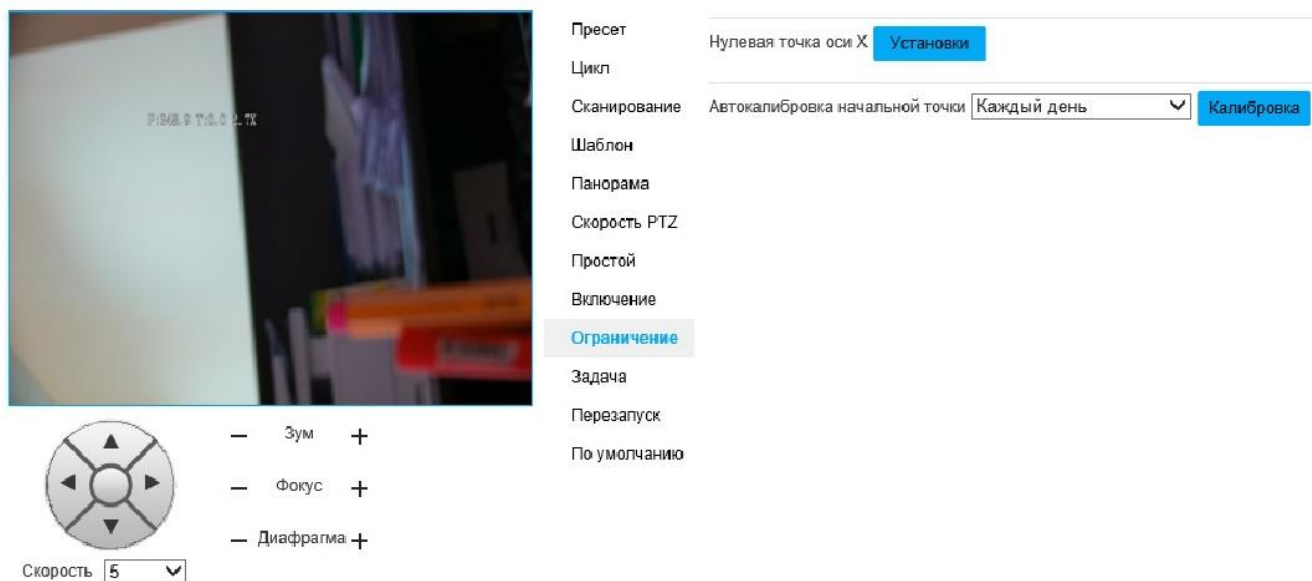
Рисунок 56 - Вкладка «Ограничение»
