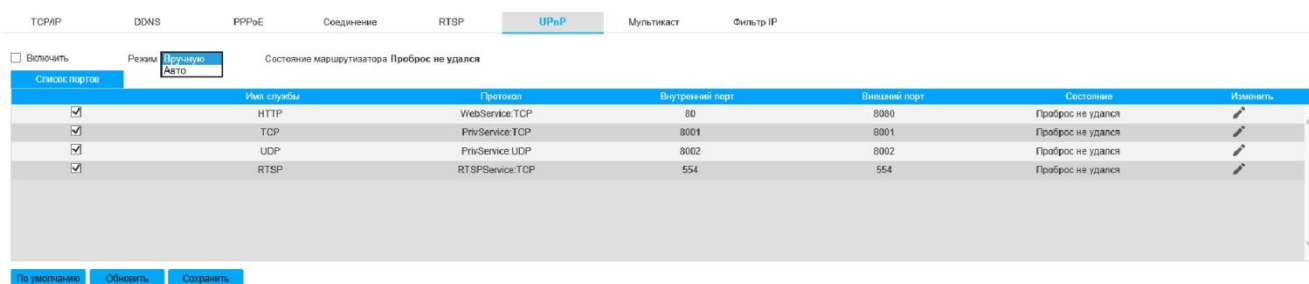
Рисунок 36 - Вкладка «UPnP»
