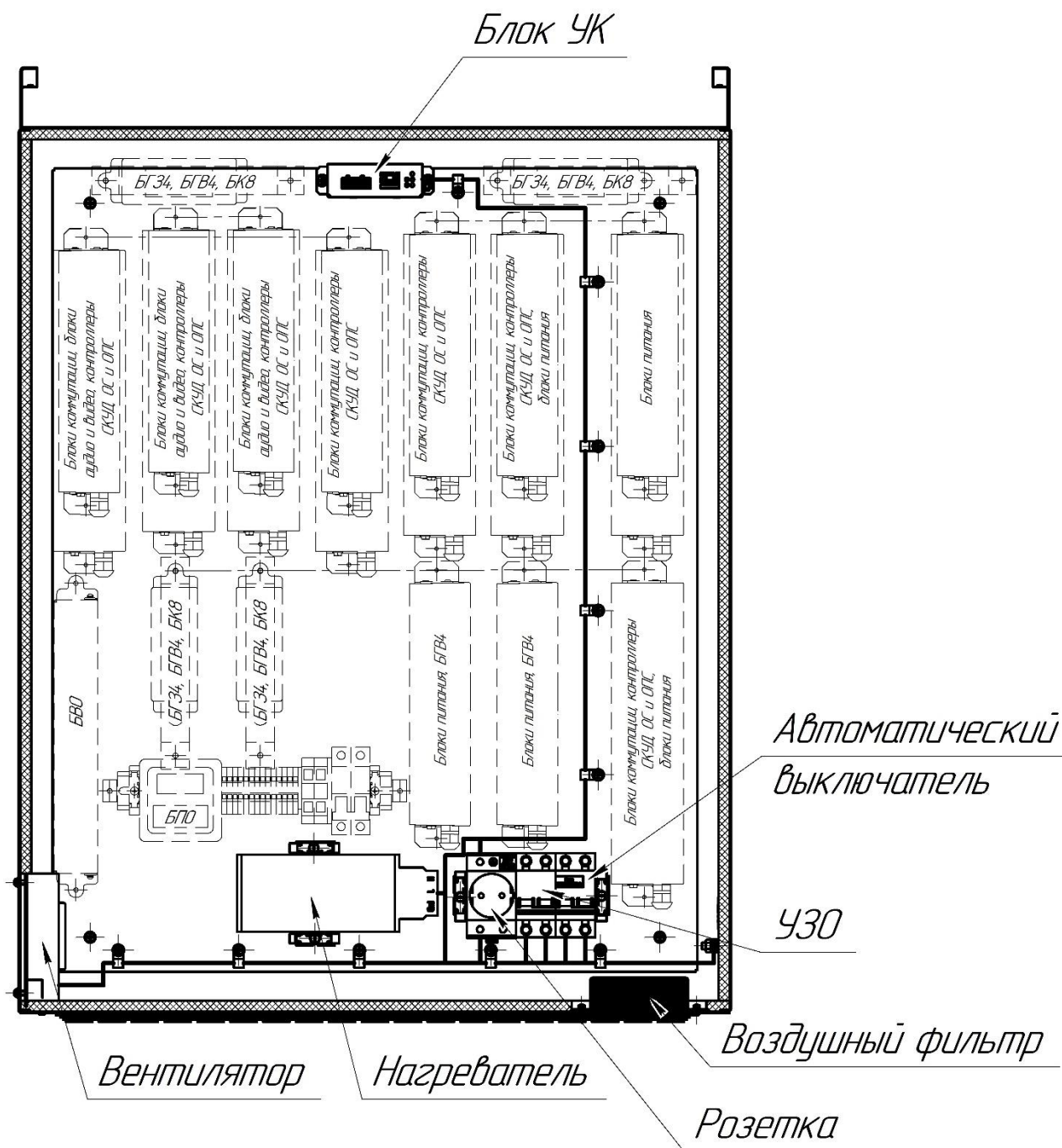
Вариант размещения блоков на монтажной панели
