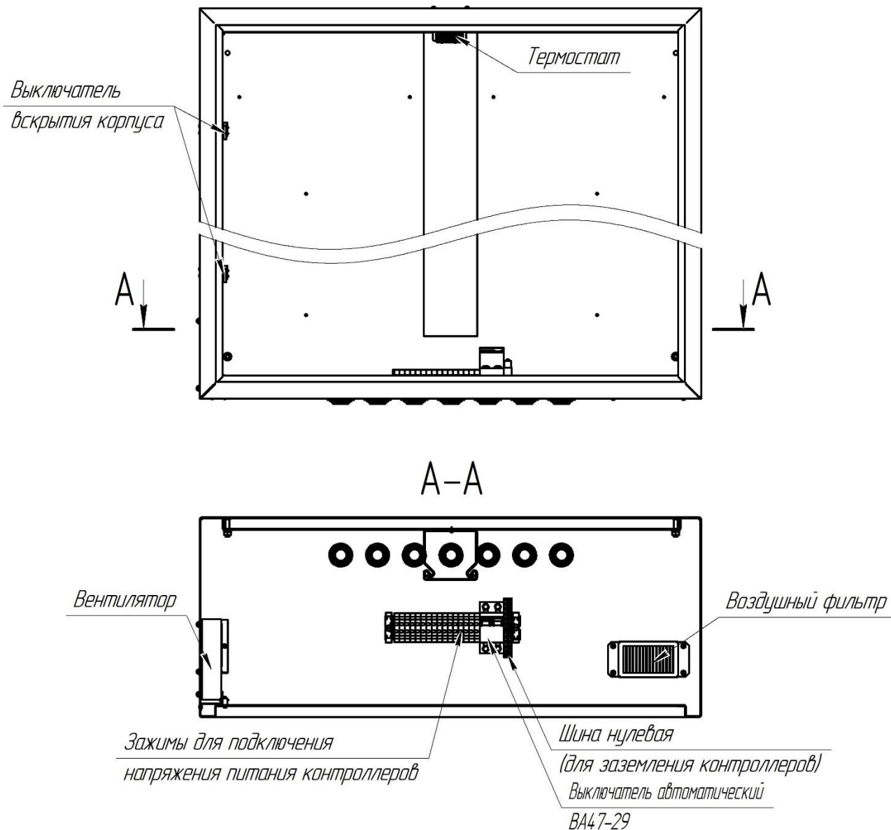
Расположение составных частей шкафа, без двери
