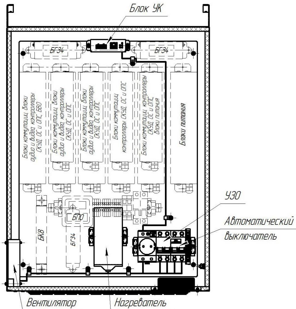
Вариант размещения блоков на монтажной панели
